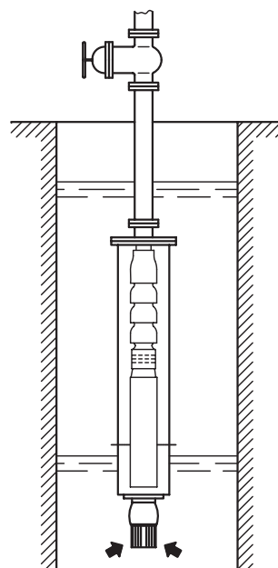
Fig. 3D Mantello aspirante verticale con valvola di fondo Picture 3D Vertical suction shell with foot valve Fig. 3D Aspiración vertical con valvula de pie Fig. 3D Jupe d'aspiration vertical avec clapet de pied Bild 3D Vertikaler Saugmantel mit Fussventil Fig. 3D Manto aspirante vertical com válvula de pé
