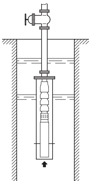
Fig. 3C Mantello aspirante verticale senza valvola di fondo Picture 3C Vertical suction shell without foot valve Fig. 3C Aspiración vertical sin valvula de pie Fig. 3C Jupe d'aspiration vertical sans clapet de pied Bild 3C Vertikaler Saugmantel ohne Fussventil Fig. 3C Manto aspirante vertical sem válvula de pé
